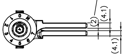
關門至0度，兩葉片尚未接觸
